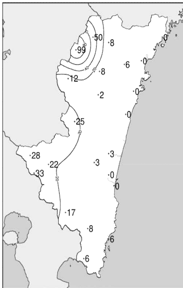
2024年12月下旬降水量平年比 (%)
