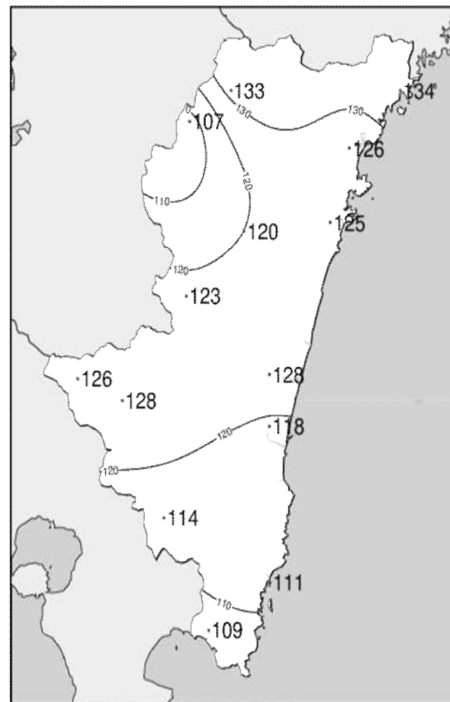
2024年12月下旬日照時間平年比 (%)
