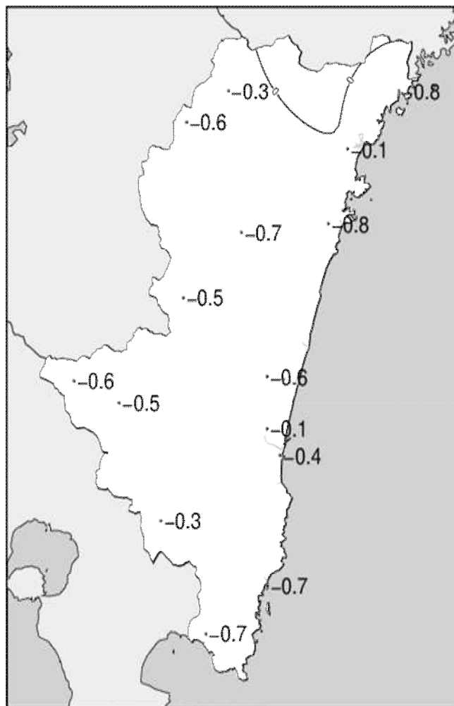
2024年12月下旬気温平年差 (°C)
