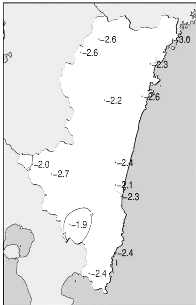
2023年1月下旬気温平年差(°C)
