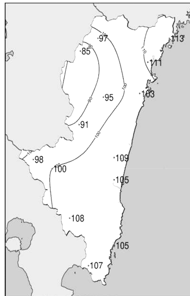
2023年1月下旬日照時間平年比(%)
