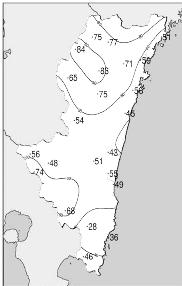
2023年1月下旬降水量平年比(%)
