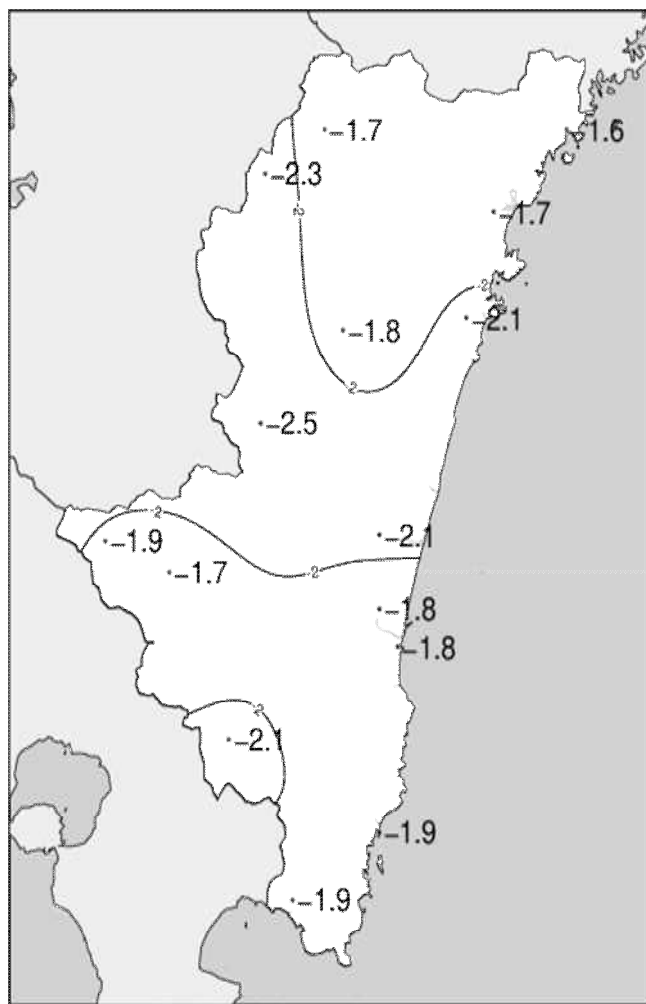
2022年12月下旬気温平年差(°C)
