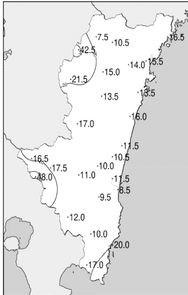
2022年12月下旬降水量観測値(ミリ)
