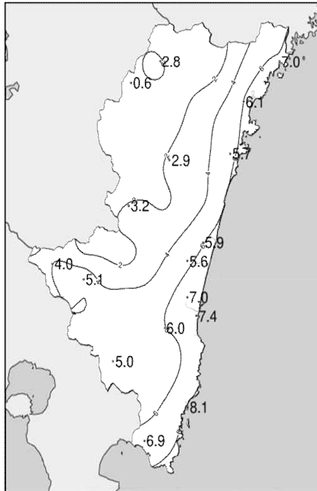
2022年12月下旬気温観測値(°C) メッシュ平年値補正
