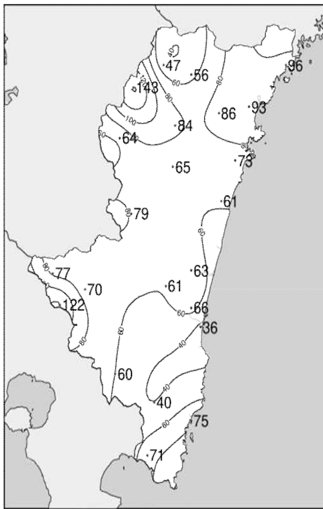
2022年12月下旬降水量平年比(%)
