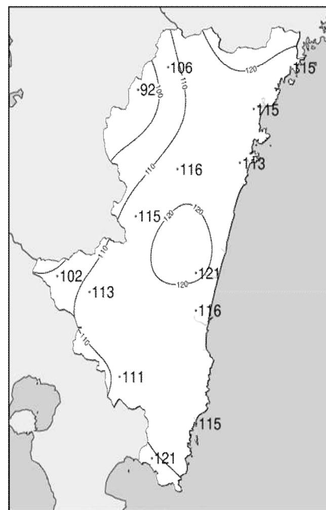
2022年12月下旬日照時間平年比(%)
